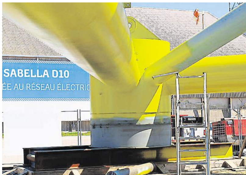
L'assemblage de l'hydrolienne se poursuit à Brest.
